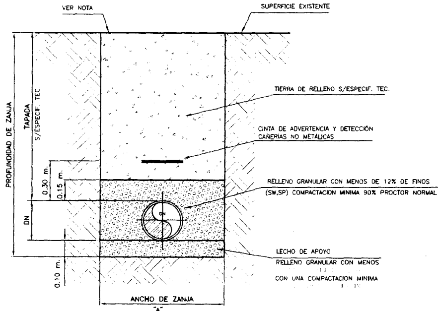
ANCHO DE ZANJA
