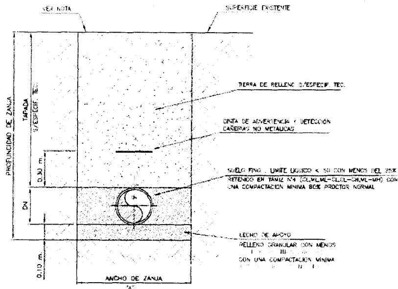
ANCHO DE ZANJA
