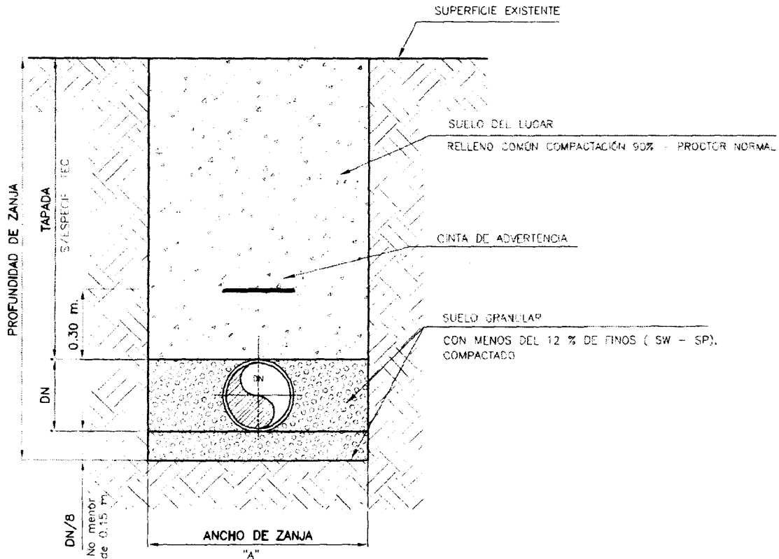
ANCHO DE ZANJA
