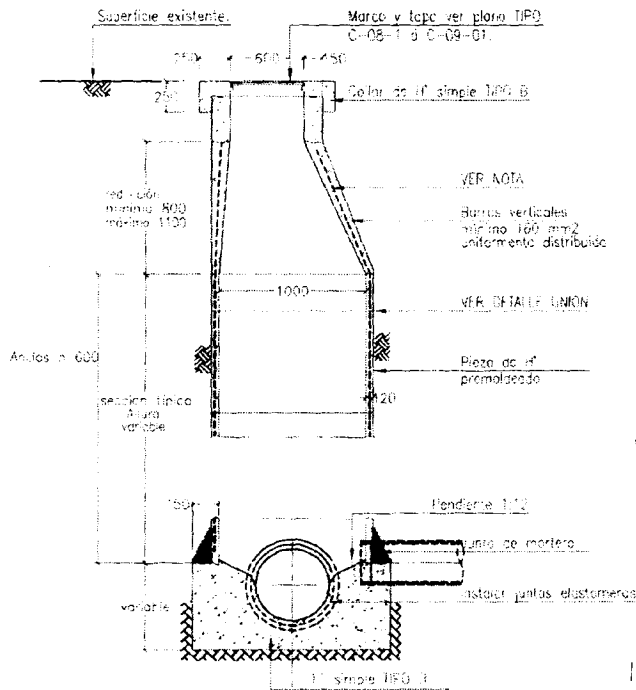
DETALLE ANILLOS PREMOLDEADOS
