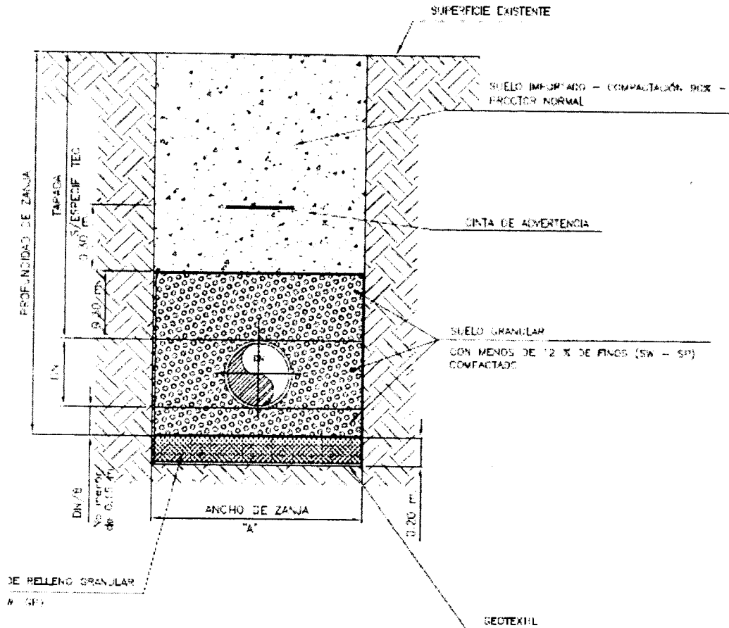
ANCHO DE ZANJA
