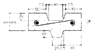
DETALLE ANILLOS PREMOLDEADOS
