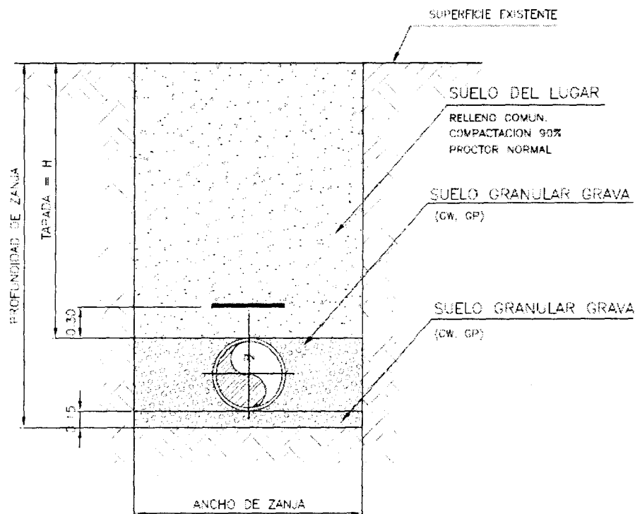
ANCHO DE ZANJA
